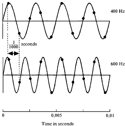
Рис. 19. Две синусоиды — с частотой 400 Гц (вверху) и 600 Гц (внизу), оцифрованные с частотой дискретизации 1000 Гц.
