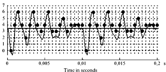
Рис. 20. Волна, оцифрованная с частотой дискретизации 5000 Гц и с 8-ю уровнями амплитуды.
