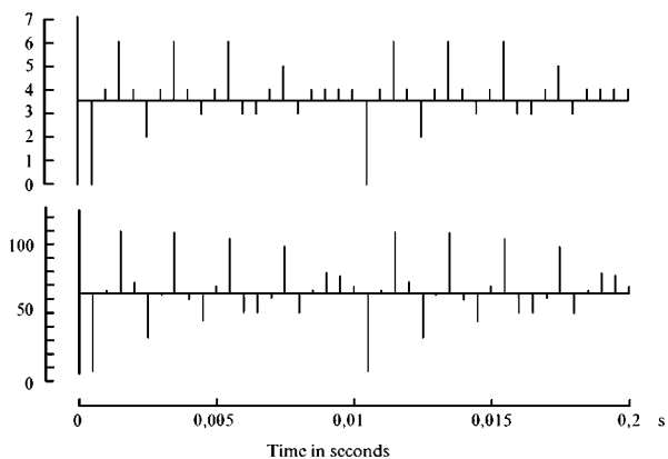
Рис. 21. Та же волна, что и на рис. 20, оцифрованная с 8-ю (вверху) и 128-ю (внизу) уровнями амплитуды
