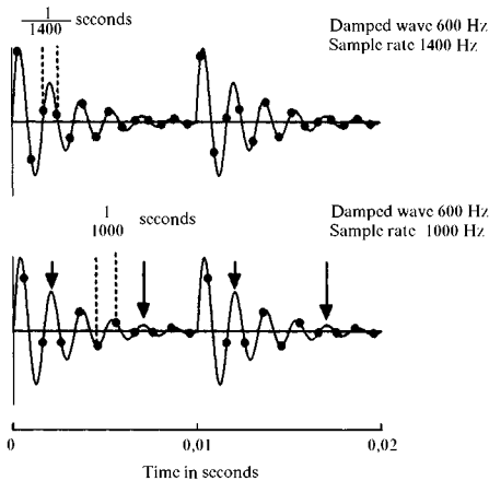
Рис. 18. Сигнал, который содержит частоту 600 Гц, оцифрованный с частотой дискретизации 1400 Гц (вверху) и 1000 Гц (внизу)
