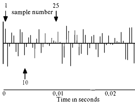
Рис. 17. Та же осциллограмма, что и на рисунке Б16, представленная с частотой дискретизации 2500 Гц
