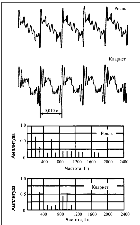
Рис. 20. Сложные периодические колебания (вверху) и их амплитудно-частотные спектры (внизу)
