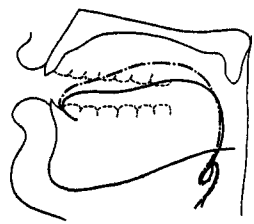
— [а] после твердого согласного - - - [а] после мягкого согласного
