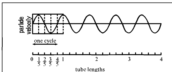
Рис. 28. Изменения скорости воздушного потока внутри трубки в \frac{5}{4} полного цикла
