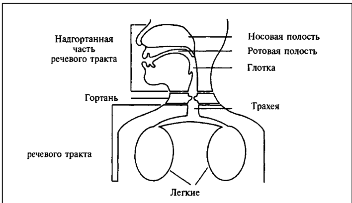
Рис. 1. Базовые компоненты речеобразующего механизма
