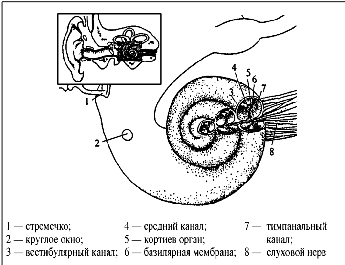
Рис. 36. Схематическое изображение строения внутреннего уха
