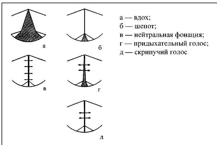
Рис. 6. Основные конфигурации глоттиса
