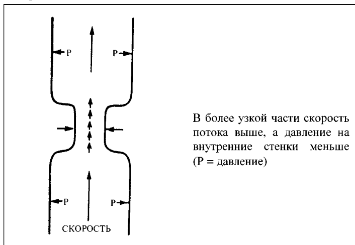
Рис. 7. Схематическое изображение воздушного потока через сужение
