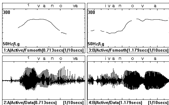
Рис. 4. Вверху — иктограмма, внизу — осциллограмма фразы Иванова, произнесенной с ИК-5 (слева) и ИК-6 (справа)
