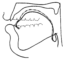
— [э] после твердого согласного - - - [е] после мягкого согласного
