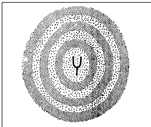
Рис. 15. Звуковые волны, распространяющиеся от источника звука
