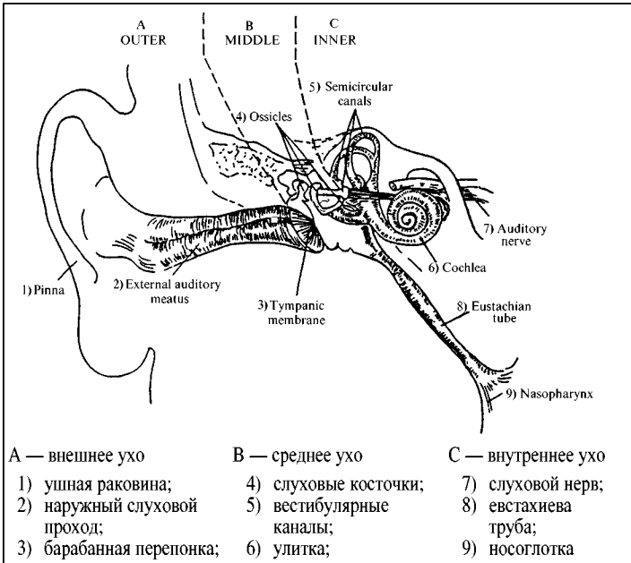
Рис. 34. Наружное, среднее и внутреннее ухо
