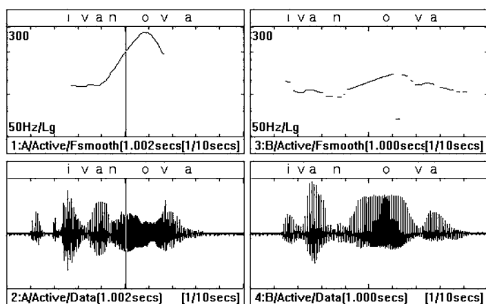
Рис. 2. Вверху — интонограмма, внизу — осциллограмма фразы Иванова, произнесенной с ИК-3 (слева — общий вопрос, справа — незавершенность)
