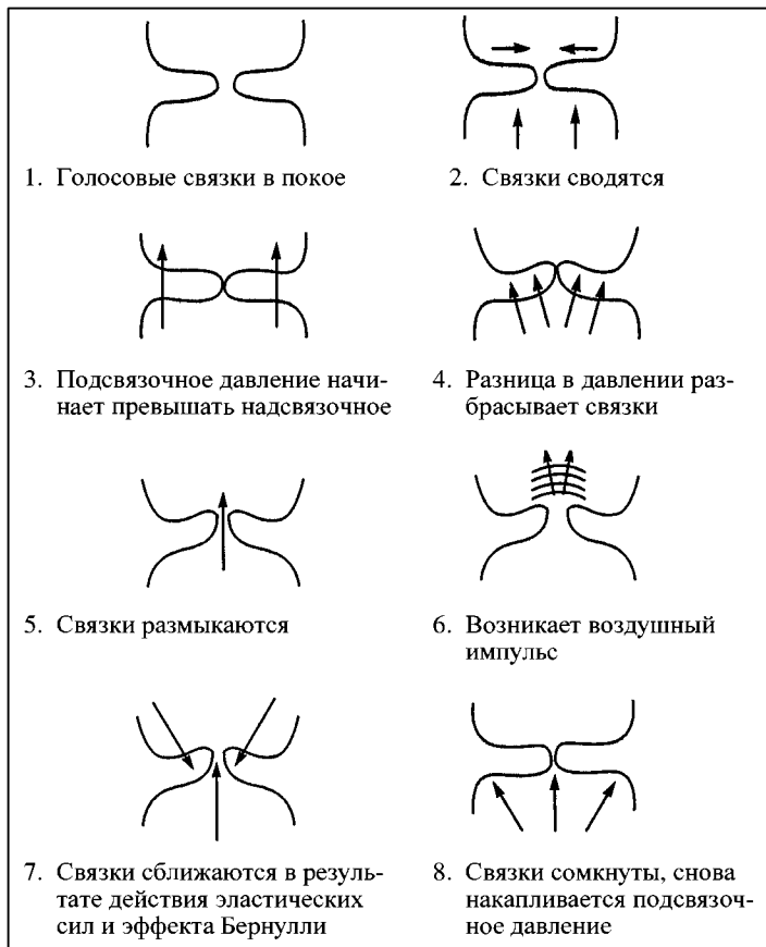
Рис. 8. Последовательные стадии колебательного цикла голосовых связок
