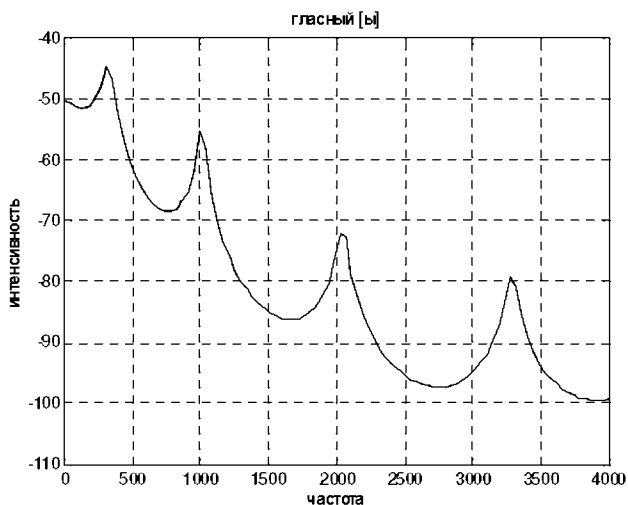
Рис 6 Спектральный срез начальной фазы гласного [ы]
