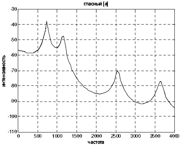
Рис 3 Спектральный срез гласного [а]
