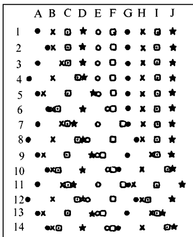
Рис. 14. Схематическое изображение десяти частиц воздуха в 14 разных моментов времени
