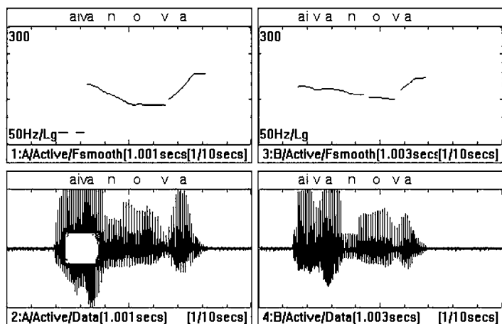
Рис. 3. Вверху — иктограмма, внизу — осциллограмма фразы А Иванова?, произнесенной с двумя разновидностями ИК-4
