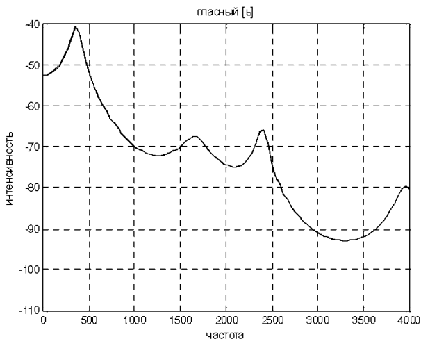
Рис 9 Спектральный срез гласного [ы]
