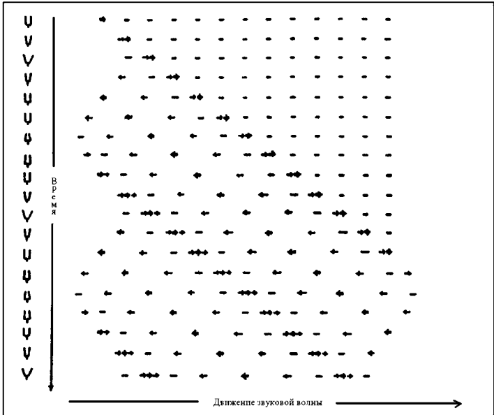
Рис. 13. Распространение звуковых волн
