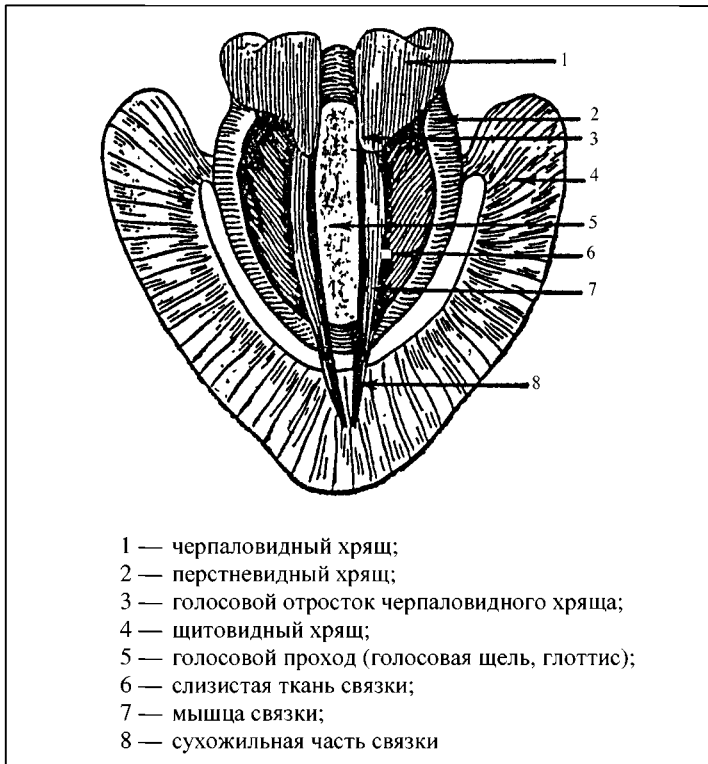
Рис. 5. Поперечный разрез гортани
