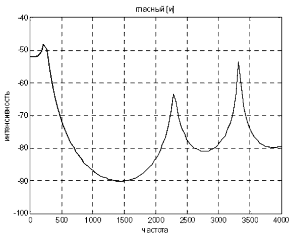
Рис 1 Спектральный срез гласного [и]
