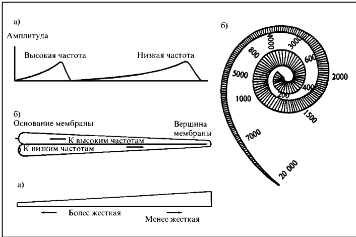
Рис. 38. Физические характеристики базилярной мембраны и чувствительность ее участков к разным звуковым частотам
