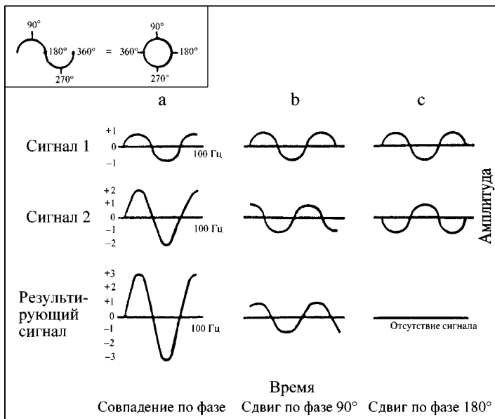
Рис. 18. Результаты взаимодействия двух гармоник (сигнал 1 и сигнал 2)
