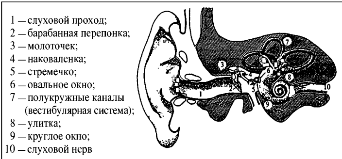
Рис. 35. Схематическое изображение слуховых органов человека
