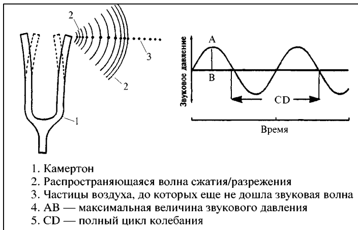
Рис. 12. Схематическое изображение изменений воздушногo давления, вызванных вибрацией камертона
