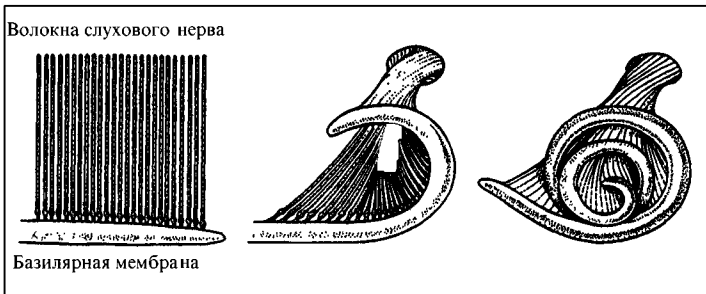
Рис. 39. Схематическое изображение связи базилярной мембраны с мозгом с помощью волокон слухового нерва
