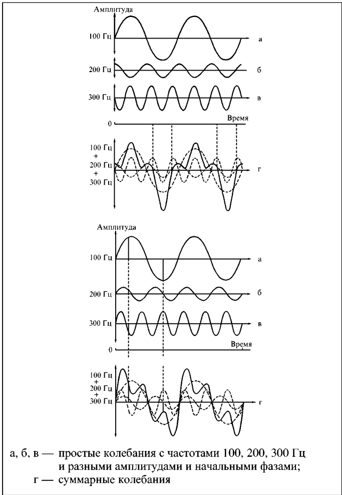
Рис. 19. Сложные периодические колебания как результат сложения простых колебаний
