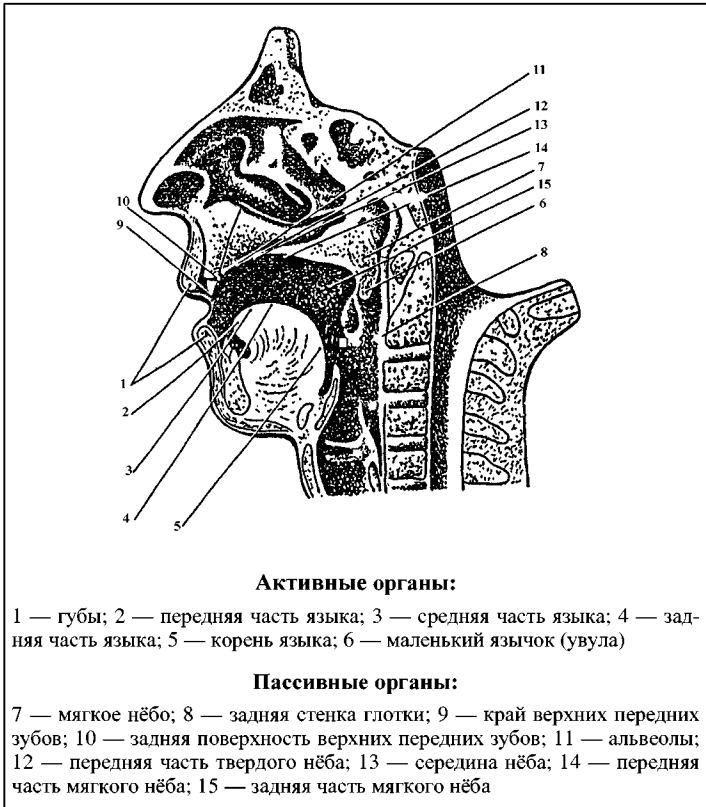
Рис. 2. Сагиттальный разрез головы
