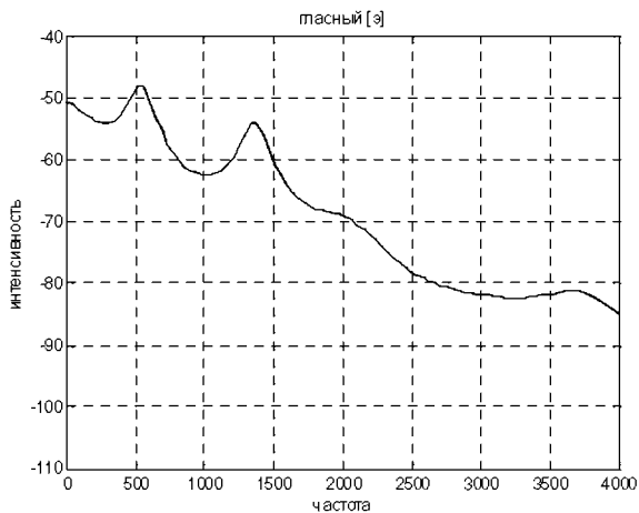
Рис 2 Спектральный срез гласного [э]
