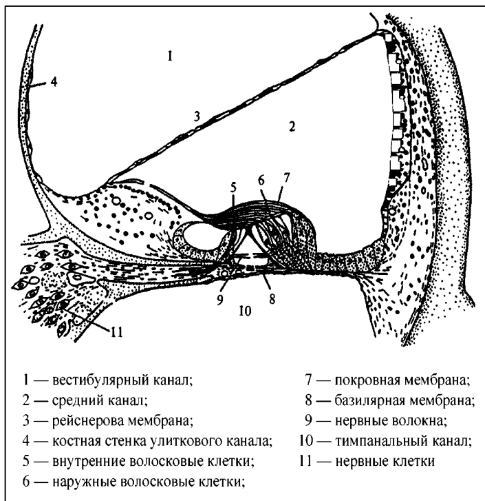
Рис. 37. Поперечный разрез улитки
