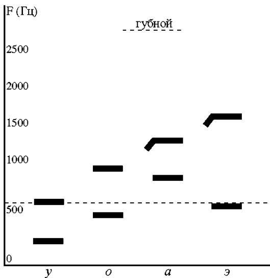
Рис 14 Формантные переходы гласных в положении после твердого губного согласного
