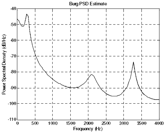
Рис 7 Спектральный срез конечной фазы гласного [ы]
