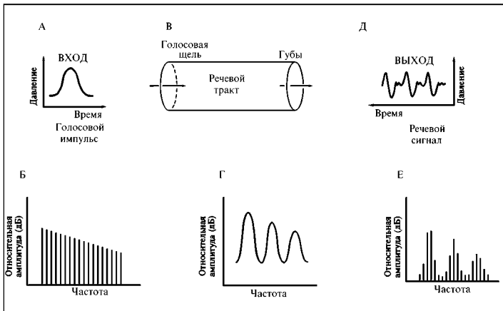
Рис. 22. Схема образования речевого сигнала при производстве гласного
