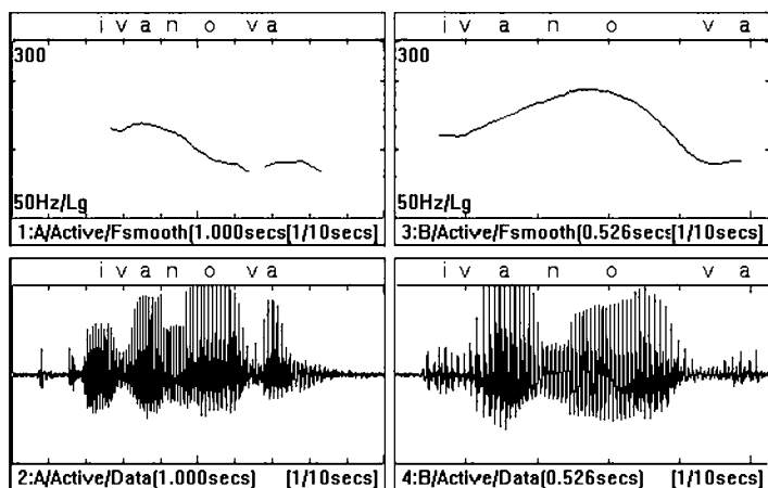
Рис. 1. Вверху — интонограмма, внизу — осциллограмма фразы Иванова, произнесенной с ИК-1 (слева) и ИК-2 (справа)
