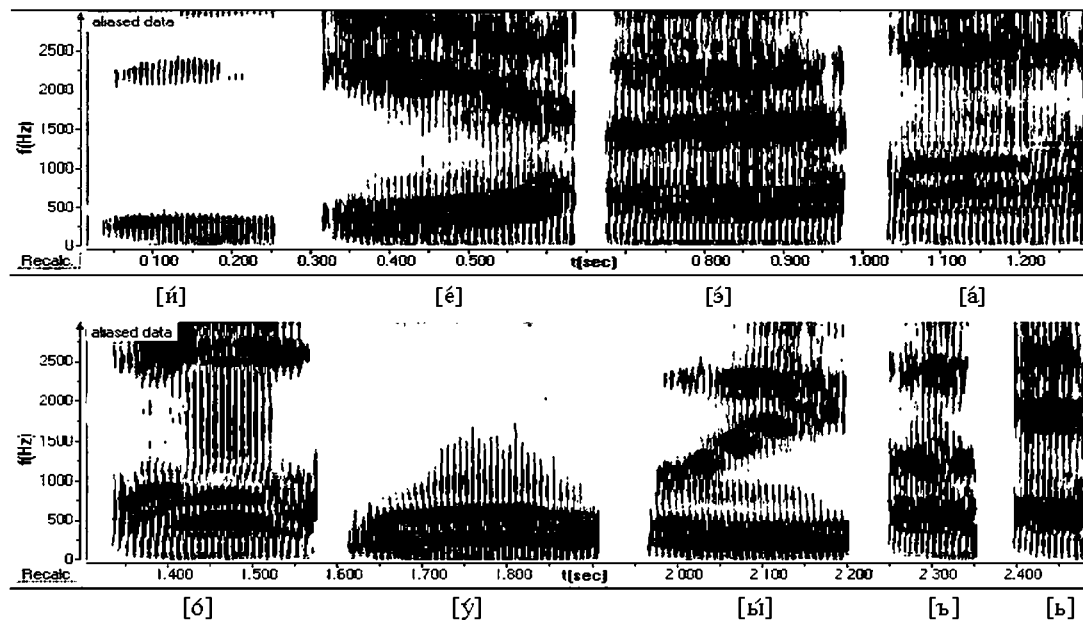
Рис. 1. Динамическая спектрограмма гласных [í], [é], [э], [á] (вверху) и [ó], [ý], [ы́], [ь], [ь] (внизу). Масштаб — до 3000 Гц
