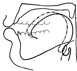
— [у] после твердого согласного - - - [у] после мягкого согласного
