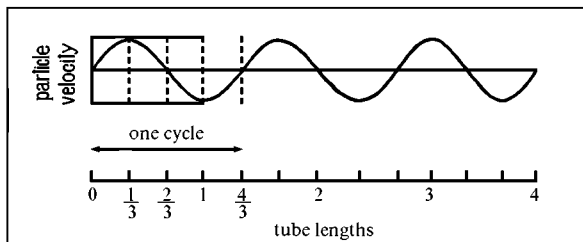
Рис. 27. Изменения скорости воздушного потока внутри трубки в \frac{3}{4} полного цикла
