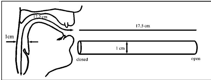
Рис. 24. Схематическое изображение речевого тракта в позиции для произнесения гласного [ʊ] и упрощенное изображение соответствующей ему формы трубки
