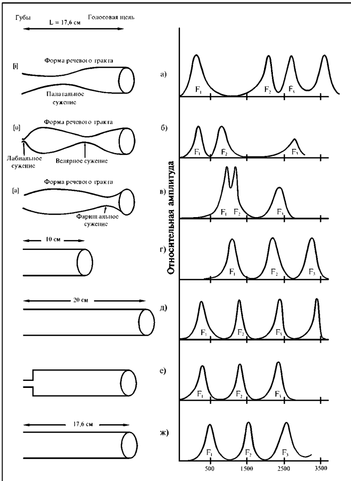
Рис. 33. Влияние формы тракта на его резонансные свойства
