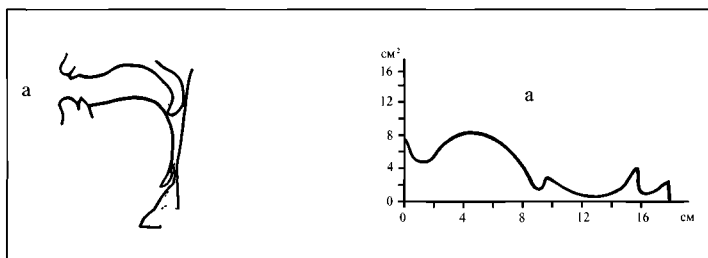
Рис. 31. Рентгенограмма (слева) и функция площади тракта (справа) для гласного [а]
