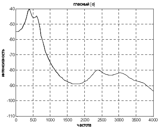
Рис 4 Спектральный срез гласного [о]
