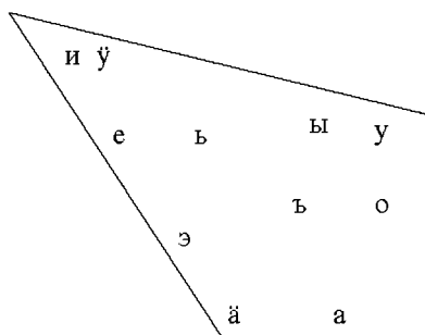
Рис 9. Трапециод гласных звуков русского языка
