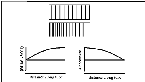
Рис. 25. Воздух в трубке, вибрирующий как пружина (вверху)
