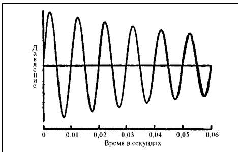
Рис. 17. Осциллограмма затухающего колебания
