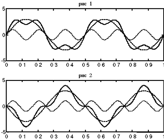
Рис 11 Различные гармоники и результирующие периодические колебания
