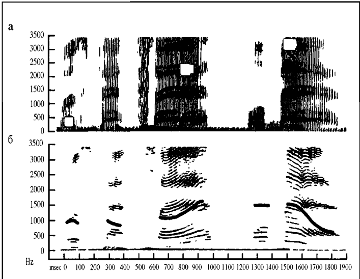
Рис. 23. Широкополосная (а) и узкополосная (б) спектрограммы
