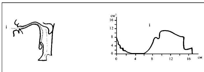
Рис. 29. Рентгенограмма (слева) и функция площади тракта (справа) для гласного [и]
