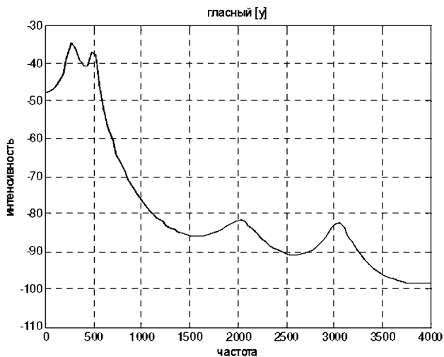
Рис 5 Спектральный срез гласного [y]
