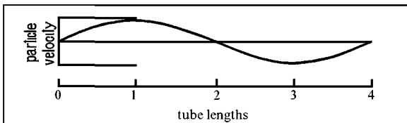
Рис. 26. График скорости воздушного потока из рис. 25, продолженный до полного цикла
