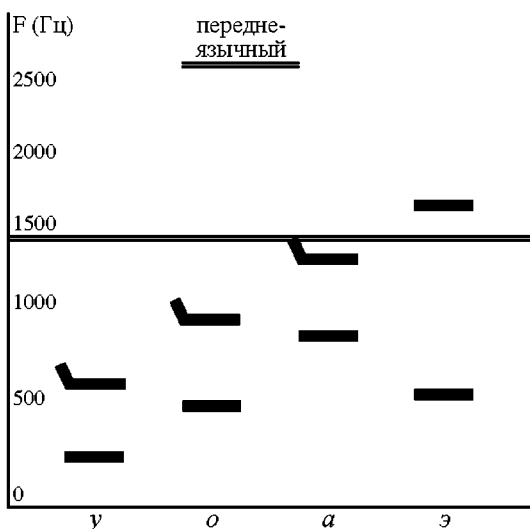
Рис 13 Формантные переходы гласных в положении после твердого переднеязычного согласного
