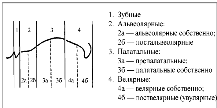
Рис. 4. Артикуляционные зоны нёба
