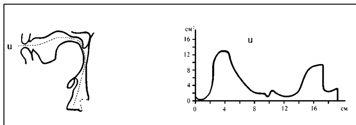
Рис. 30. Рентгенограмма (слева) и функция площади тракта (справа) для гласного [у]
