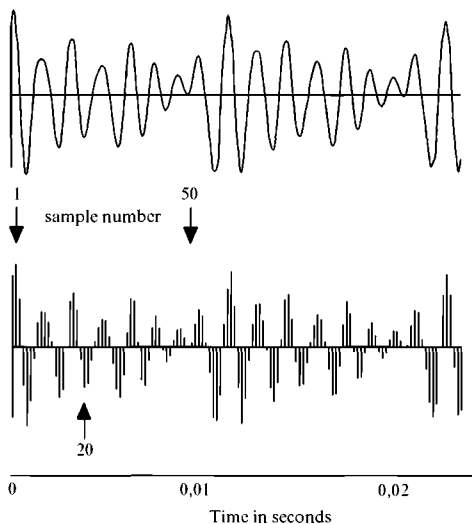
Рис. 16. Вверху — непрерывный сигнал (осциллограмма двух периодов гласного [а]), внизу — линии, соответствующие амплитуде колебаний через равные промежутки времени (цифры означают номер линии в месте стрелки). Частота дискретизации — 5000 Гц
