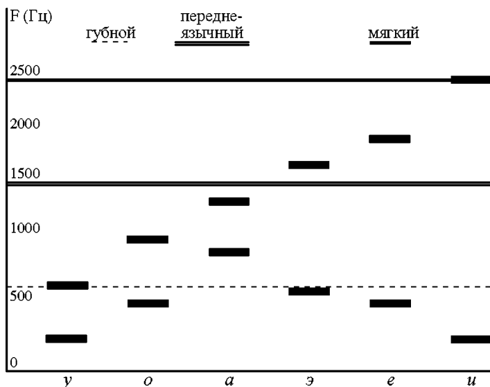
Рис 12 Приблизительные значения F_1 и F_2 русских гласных и локусы F_2 некоторых классов русских согласных
