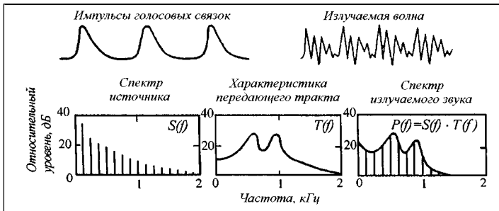
Рис. 21. Схема образования звука с голосовым источником
